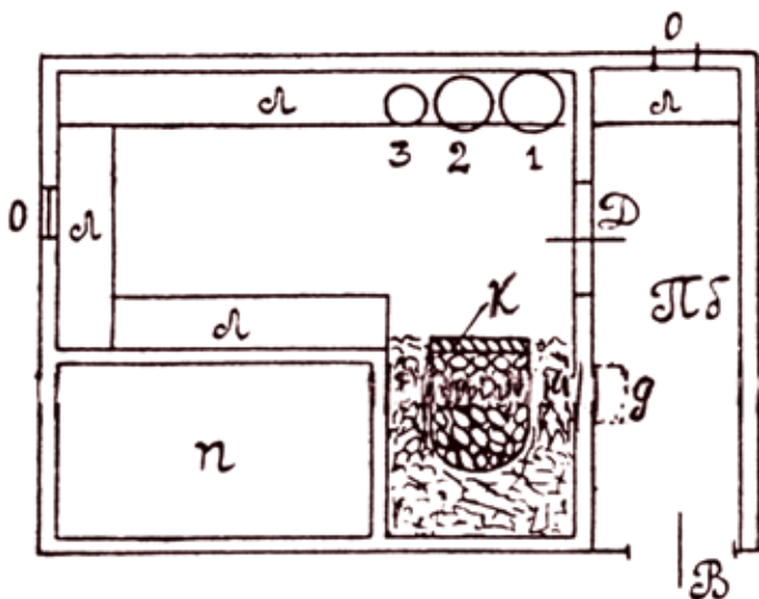
План севернорусской бани. Вологодская губ. Тотемский у.
