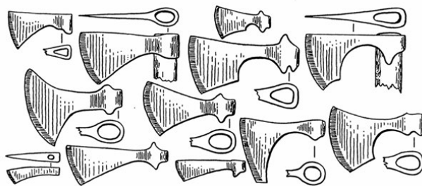
Рабочие топоры. XII–XIV вв.
