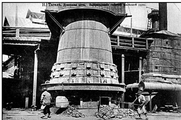
Нижний Тагил. Доменная печь. Выбрасывание горячей железной руды.
