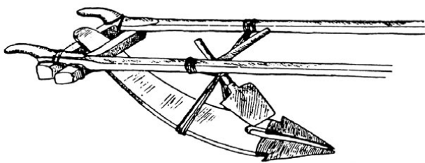
Рис. 2 Севернорусская соха с перекладной полицей. Пермская губ.
